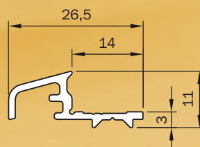
Profil odwadniający II
