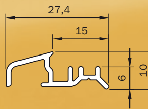
Profil odwadniający IV
